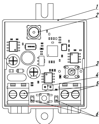
Рисунок 2 - Внутреннее устройство расширителя
