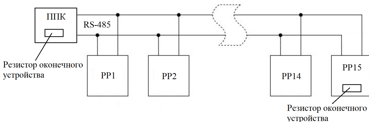
Рисунок 3 - Типовая схема подключения расширителей
