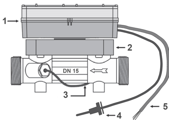
Рисунок 2 – Внешний вид счетчика ( вид сбоку)
